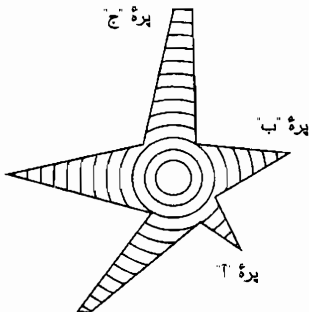
شکل ۳-۲: حرکت موج آب بر روی سطح آب حوضی به شکل یک ستاره
