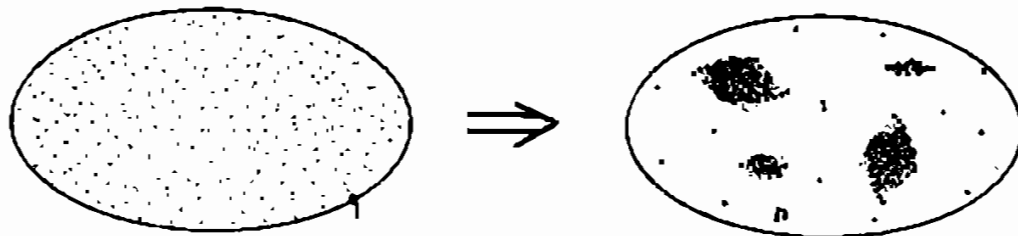
توزیع یکنواخت ستارگان
