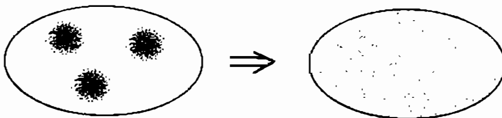
توزیع منظم مولکول‌های گاز
